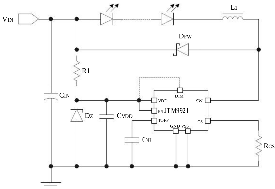
图 1: JTM9921 典型应用电路图
