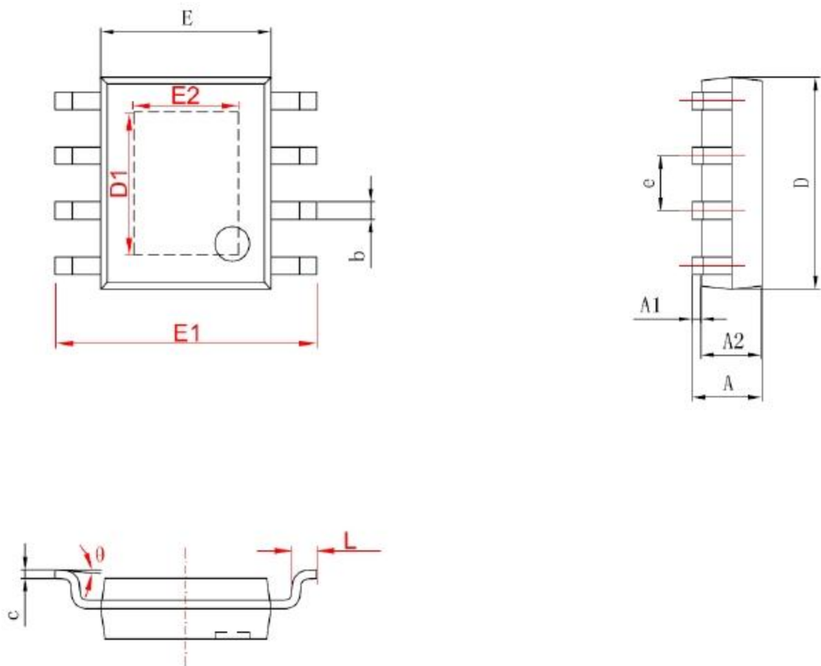
ESOP8 封装参数
