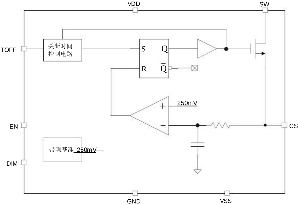
图 2: JTM9921 内部电路方框图
