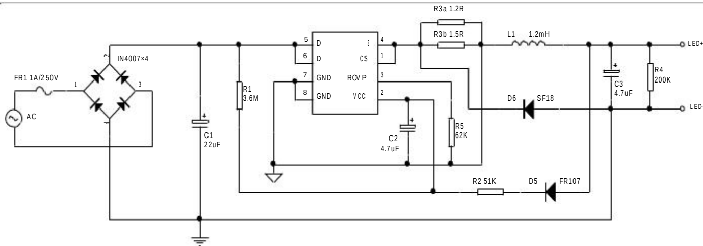
JTM9129MB-30W 典型应用电路
