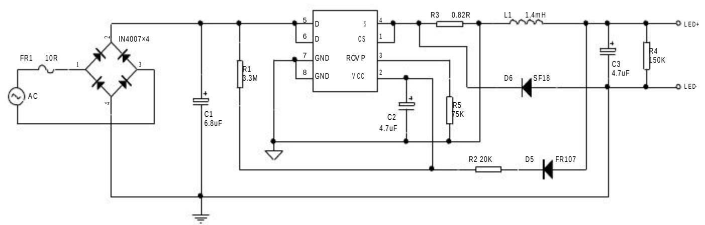
JTM9129MA-18W 典型应用电路
