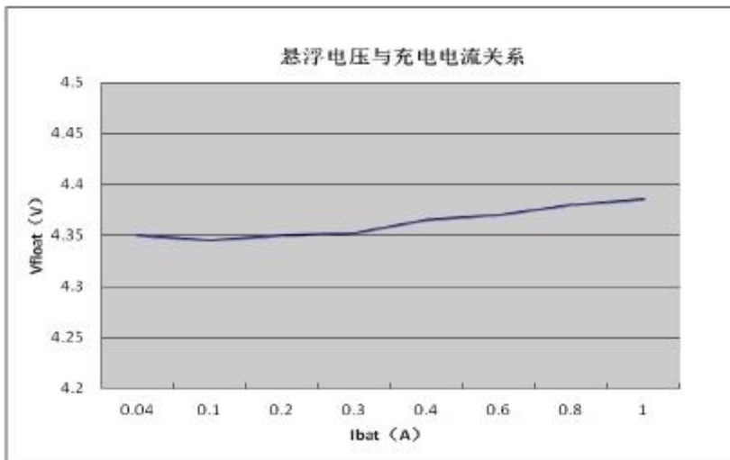
ΔFigure 14. 悬浮电压与充电电流关系图 (测试条件: VCC=5V)
