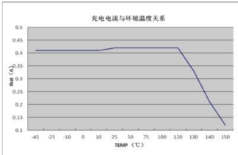
ΔFigure 13. 充电电流与环境温度关系 (VCC=5V, VBAT= 4V, RPOG=3K)
