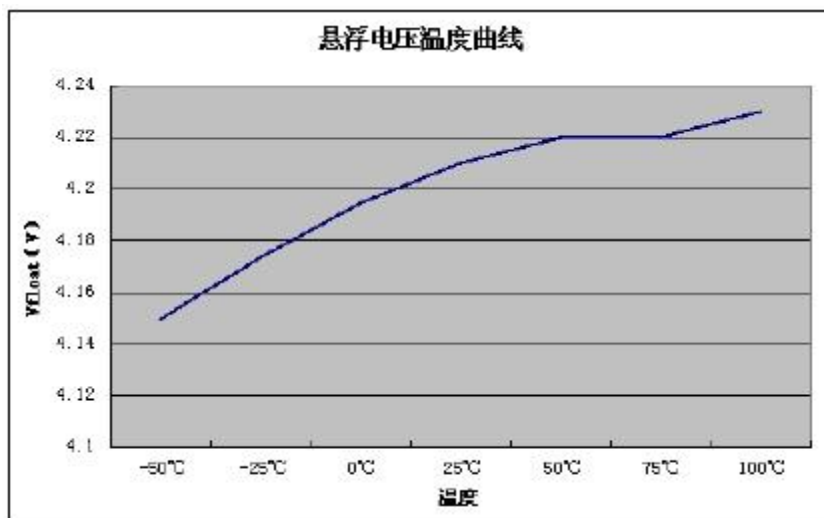
*Figure 1. 悬浮电压曲线图 (测试条件: VCC=5V, RPROG=2.4K)
