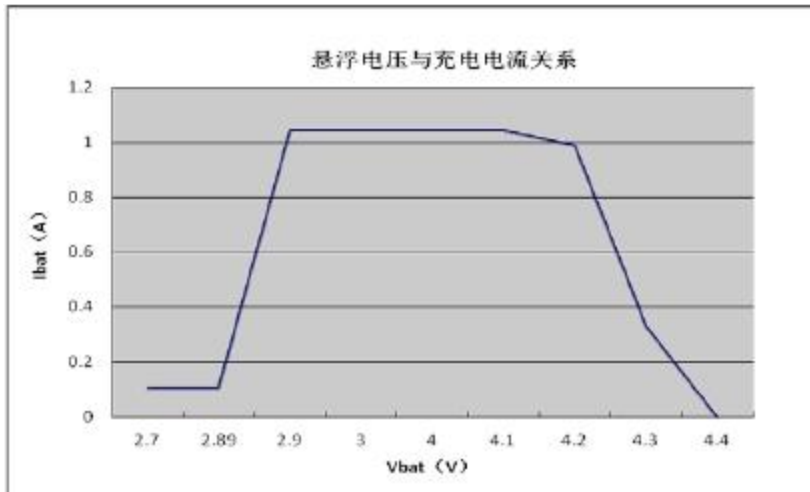
ΔFigure 15. 充电电流与电池关系图 (测试条件: VCC=5V, Rprog=1.2K)
