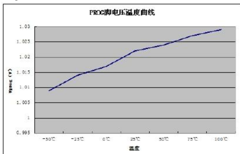
* Figure 2. PROG 脚电压温度曲线 (测试条件: VCC=5V, VBAT=3.7V, RPROG=2.4K)
