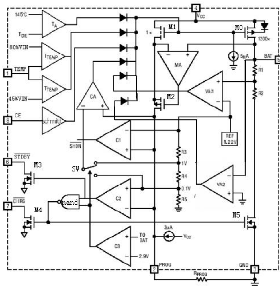
方框图
