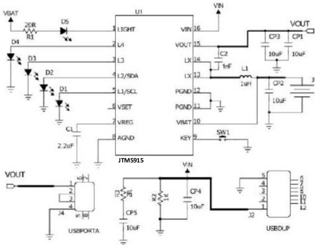
图 7 4LED 电量显示典型应用原理图
