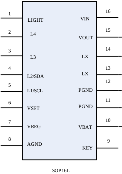
图 2 5 5 引脚图
