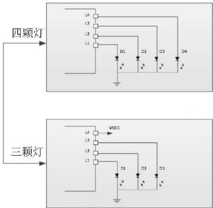
图 4 三颗、四颗灯 LED PIN 连接方式
