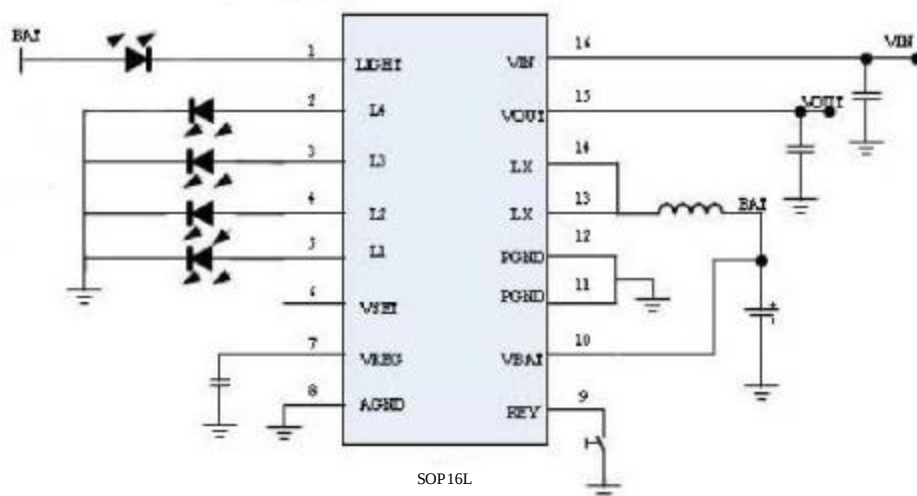
图 1 简化应用原理图(4 LED 指示电量)
