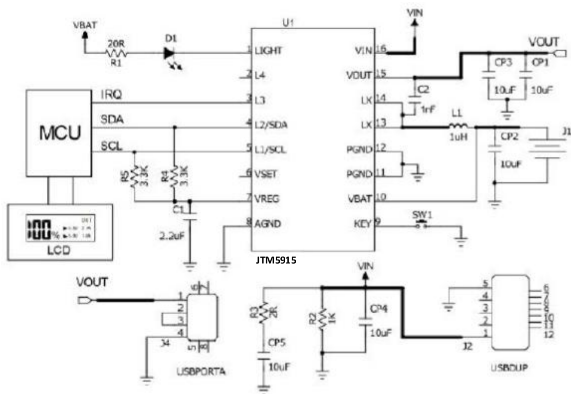
图 8 I2C 应用的典型应用原理图
