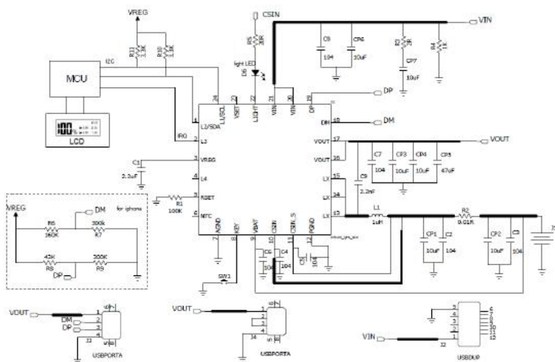
图 6 I2C 应用的典型应用原理图
