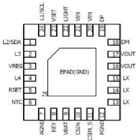
图 2 JTM5919 引脚图
