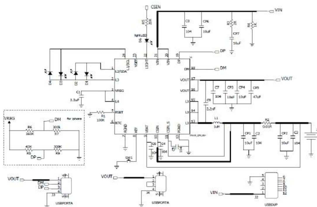
图 5 4LED 电量显示典型应用原理图
