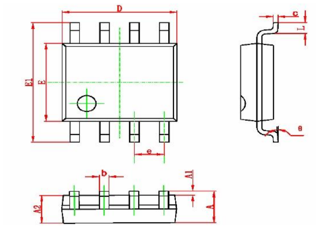
SOP8 封装外型尺寸图
