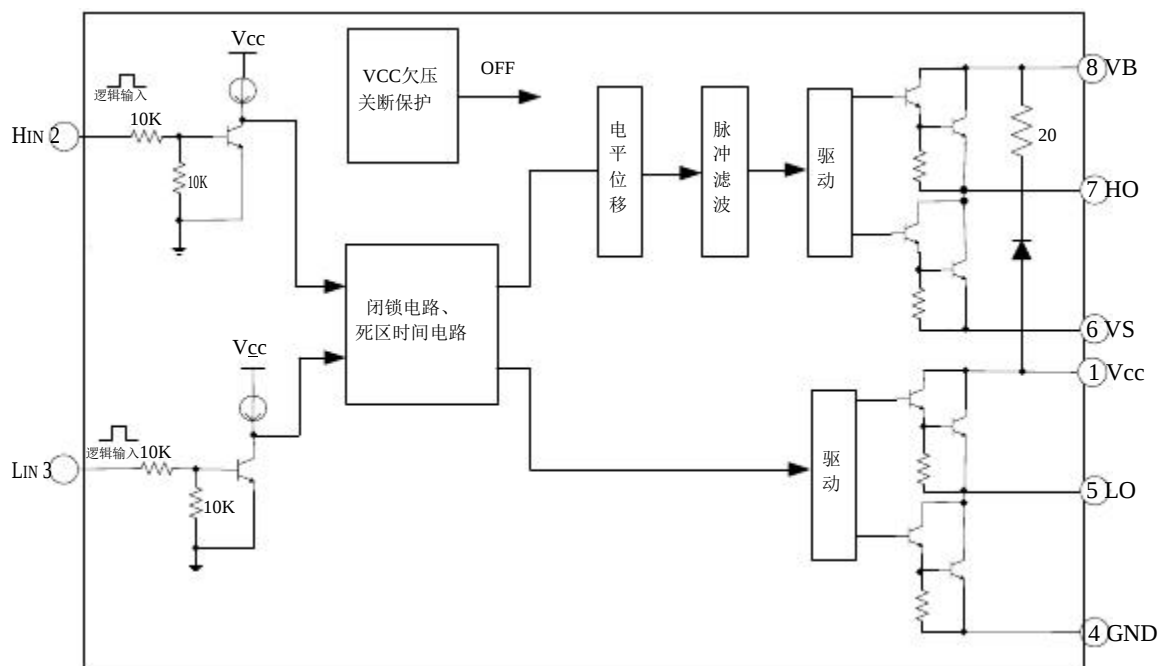
图 5-1. JTM2106 结构框图
