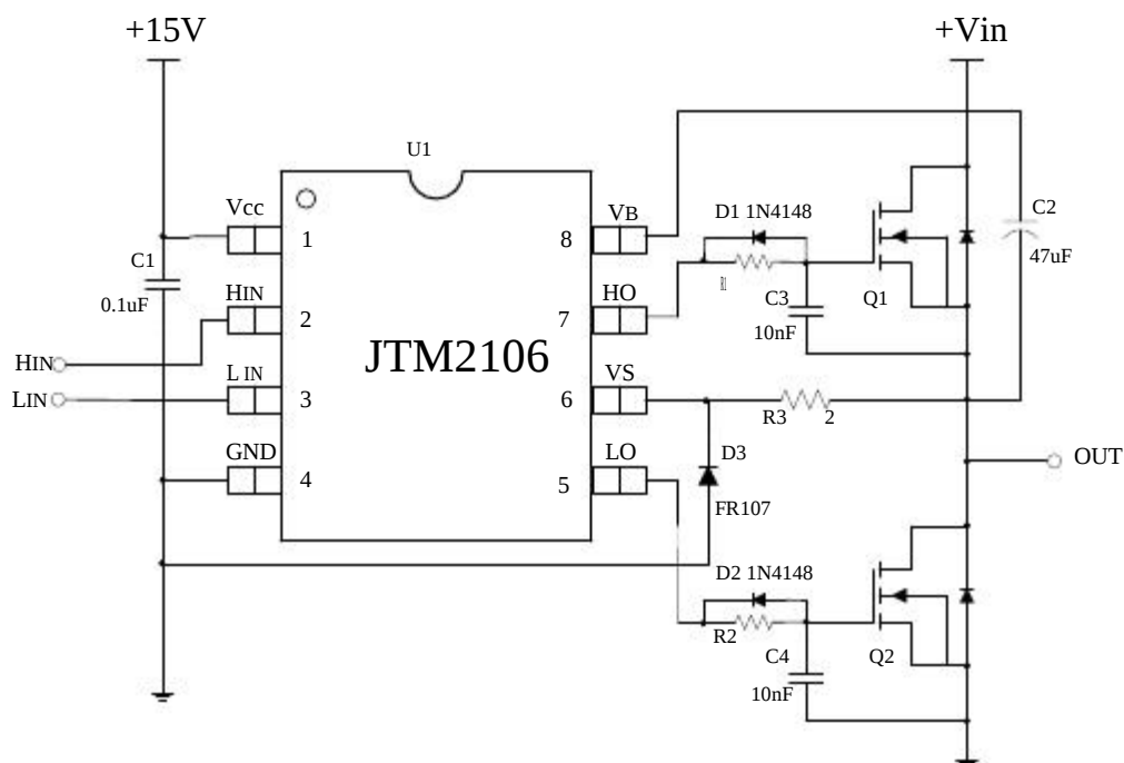
图 6-2. JTM2106 典型应用电路图——大功率电机场合应用
