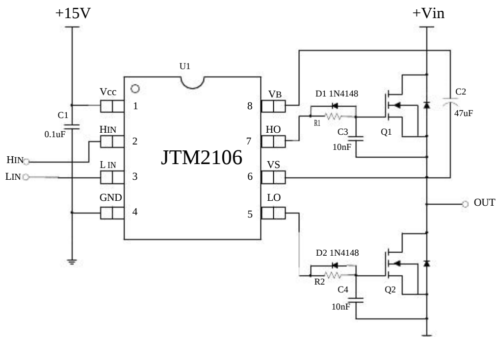
图 6-1. JTM2106 典型应用电路图——中、小功率半桥驱动应用
