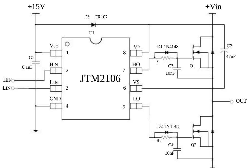
图 6-3. JTM2106 典型应用电路图——外接自举二极管应用
