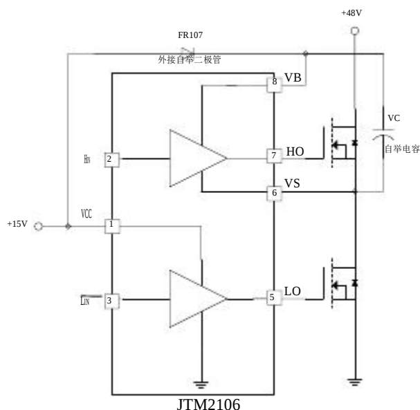
图 8-3. JTM2106 自举电路结构
