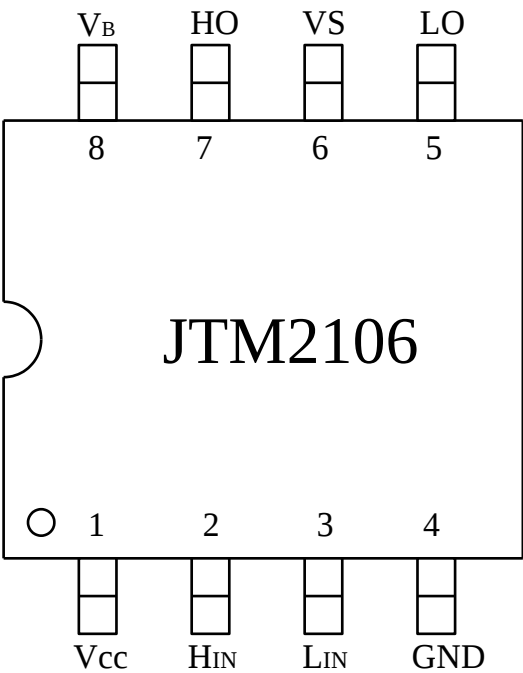
图 4-1. JTM2106 管脚定义
