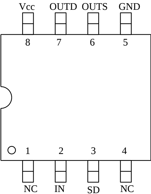
图 4-1. JTM2117 管脚定义
