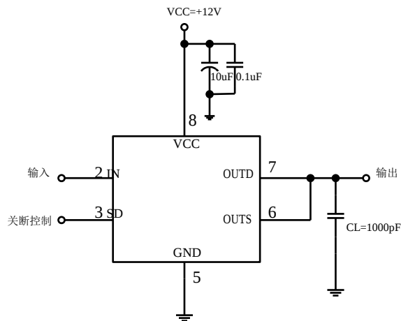
输入：100kHz 方波 Trise=Tfall≤10nS
