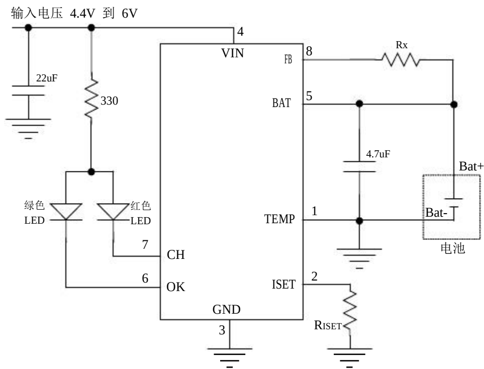
图 2 应用电路（利用外接电阻调整恒压充电电压）
