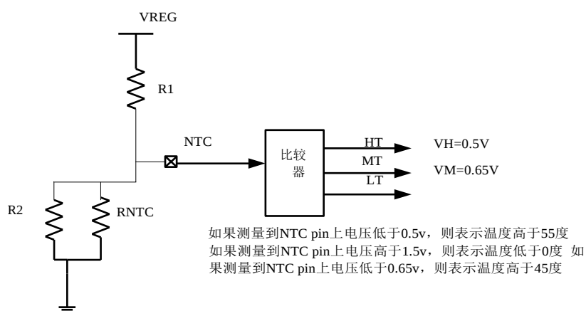
图 6 电池 NTC 比较
