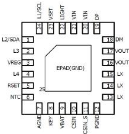
图 2 JTM5929 引脚图
