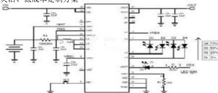
图 1 简化应用原理图(4 LED 指示电量)
