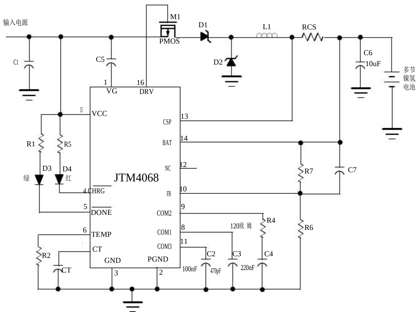
图 1 典型应用电路
