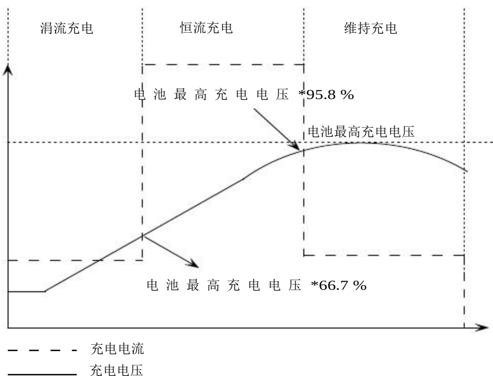
图 2 充电过程示意图
