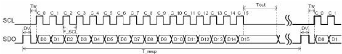
图 1.1 16 键输入，高电平有效时序
