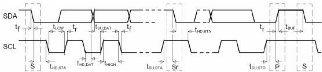
图 2.4 I2C 总线上 F/S 模式设备的时序定义
