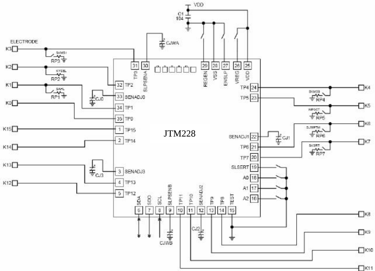
图 9-1 16 键模式参考电路图
