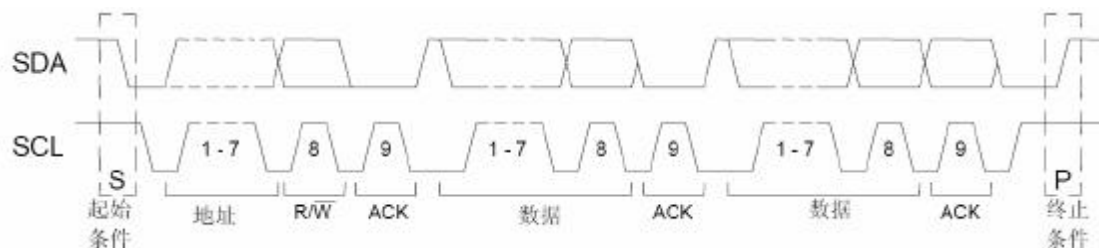
图 2.3 一次完整的数据传送
