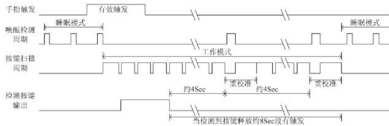
图 5-2 睡眠模式转到工作模式的时序图
