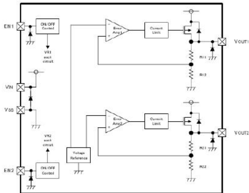
图1 9182 功能框图
