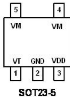
SOT23-5
