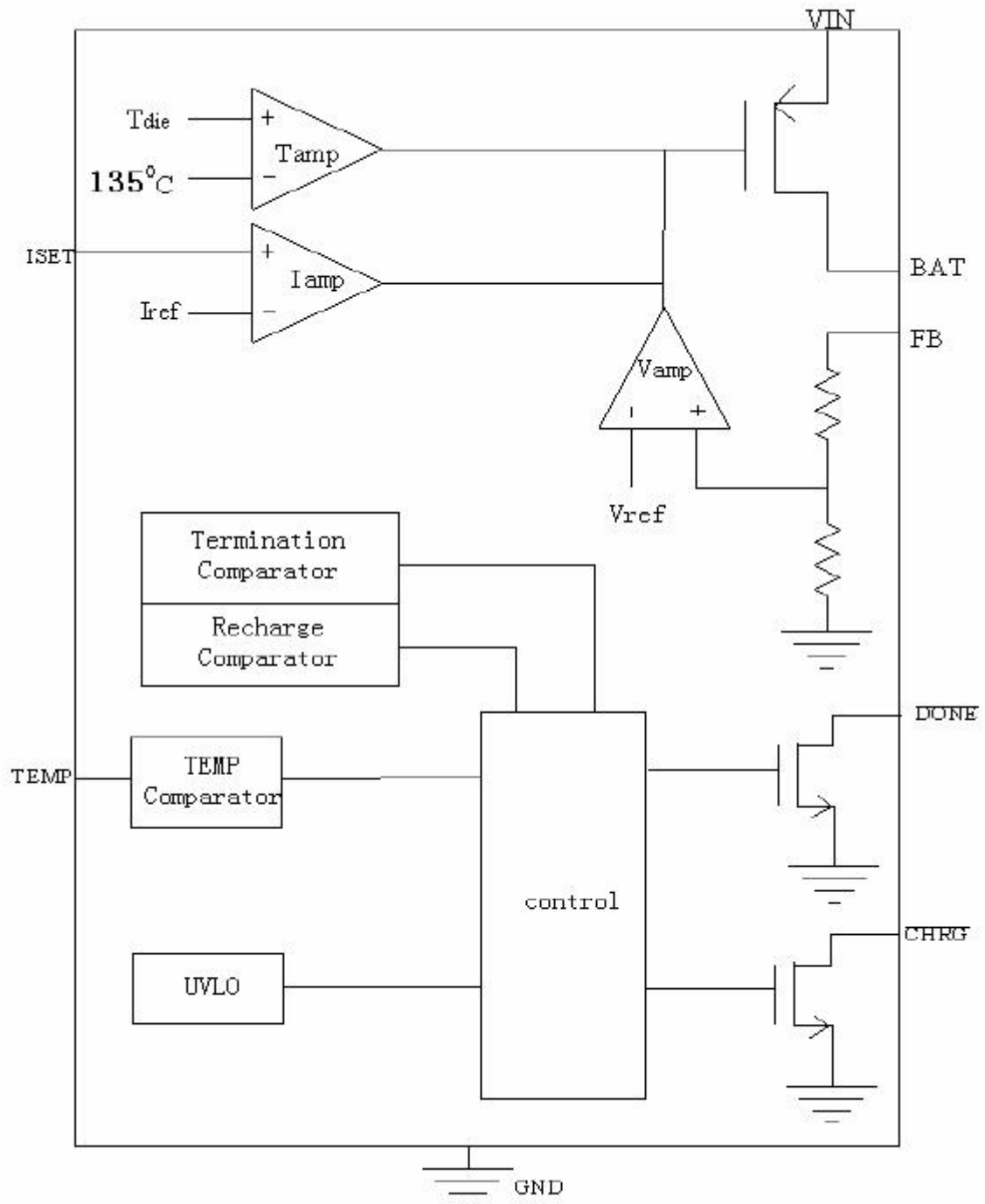
图 3 功能框图
