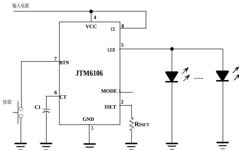
图 5 JTM6106 驱动并联发光二极管(LED)
