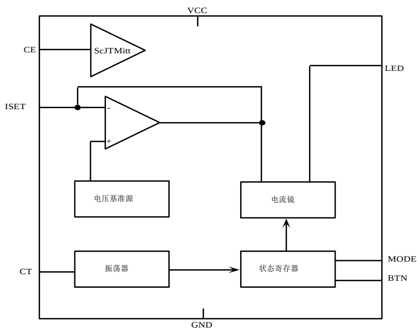
图 4 功能框图
