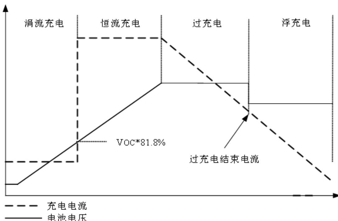
图 2 充电过程示意图
