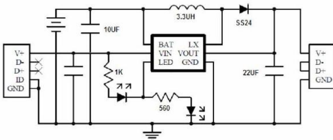
图1. JTM1605典型应用电路图
