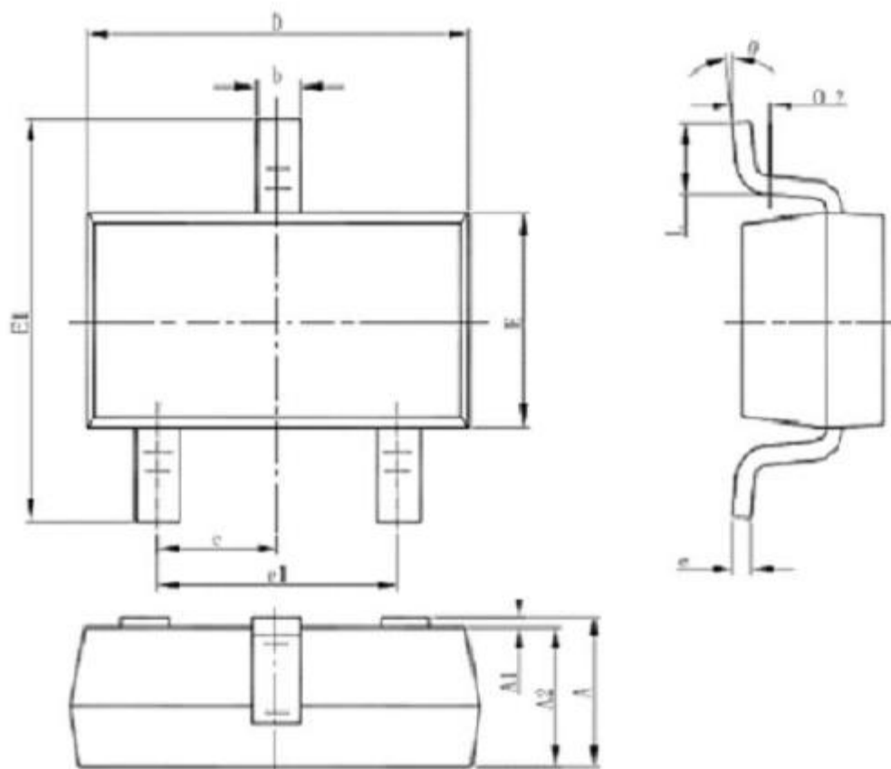
SOT-23-3
