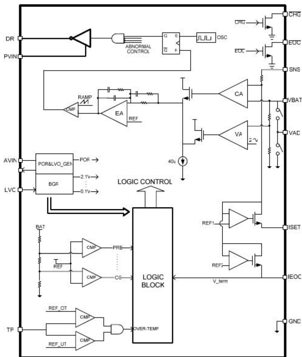
图 3. JTM4061 功能框图
