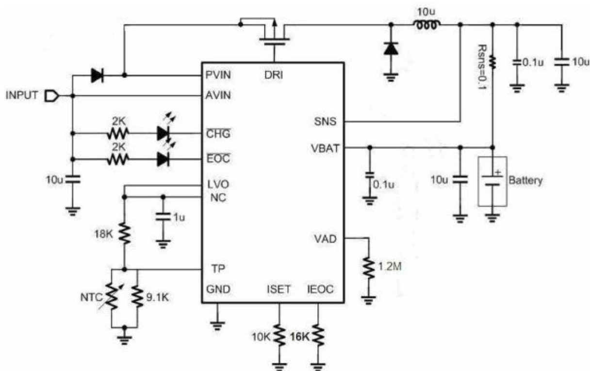
图 1.1.JTM4061 单节充电典型应用图
