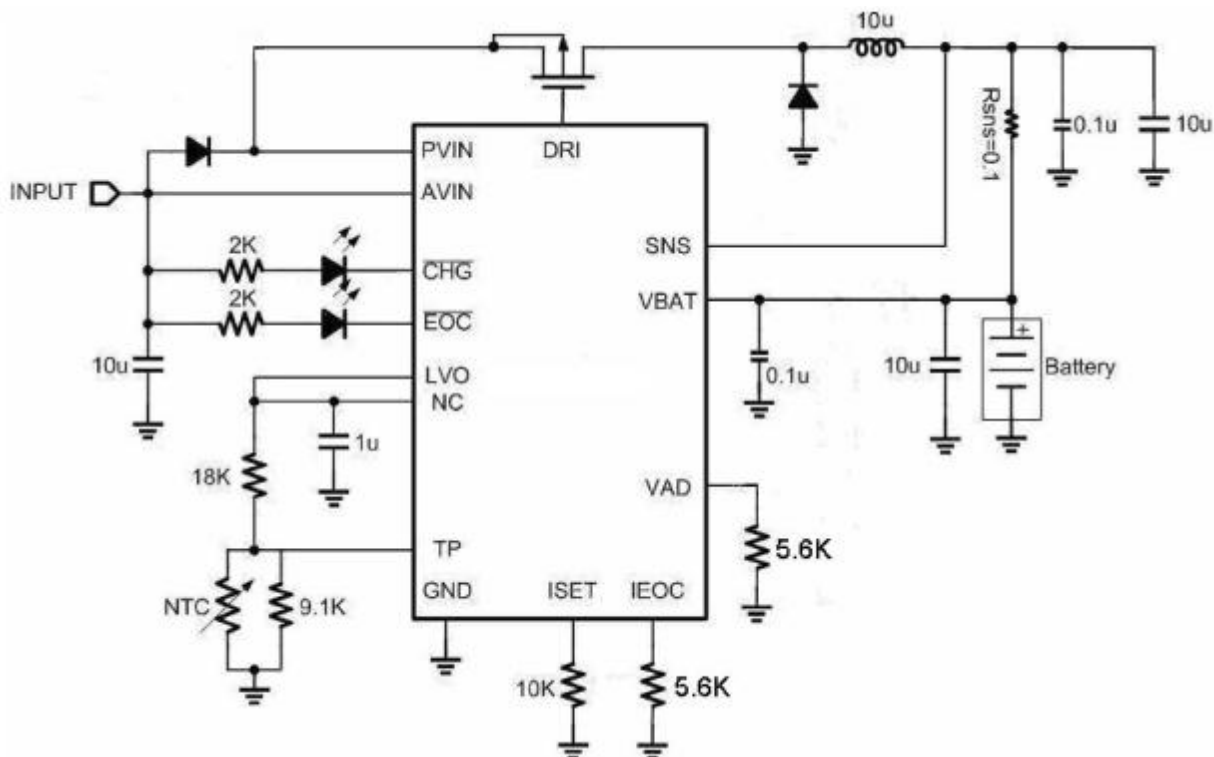
图 1.2.JTM4061 双节充电典型应用图
