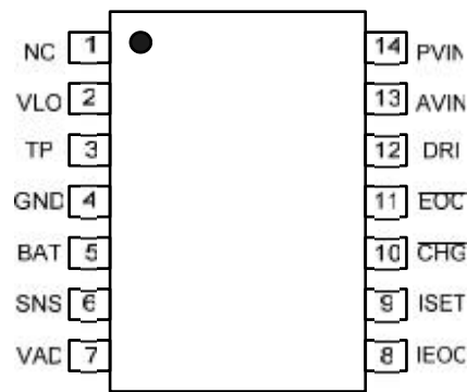
图 2. JTM4061 管脚定义
