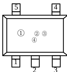
SOT-23-5L
