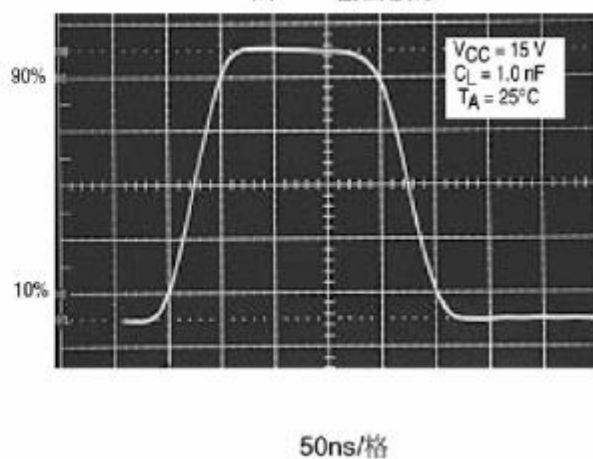
图 14. 输出波形
