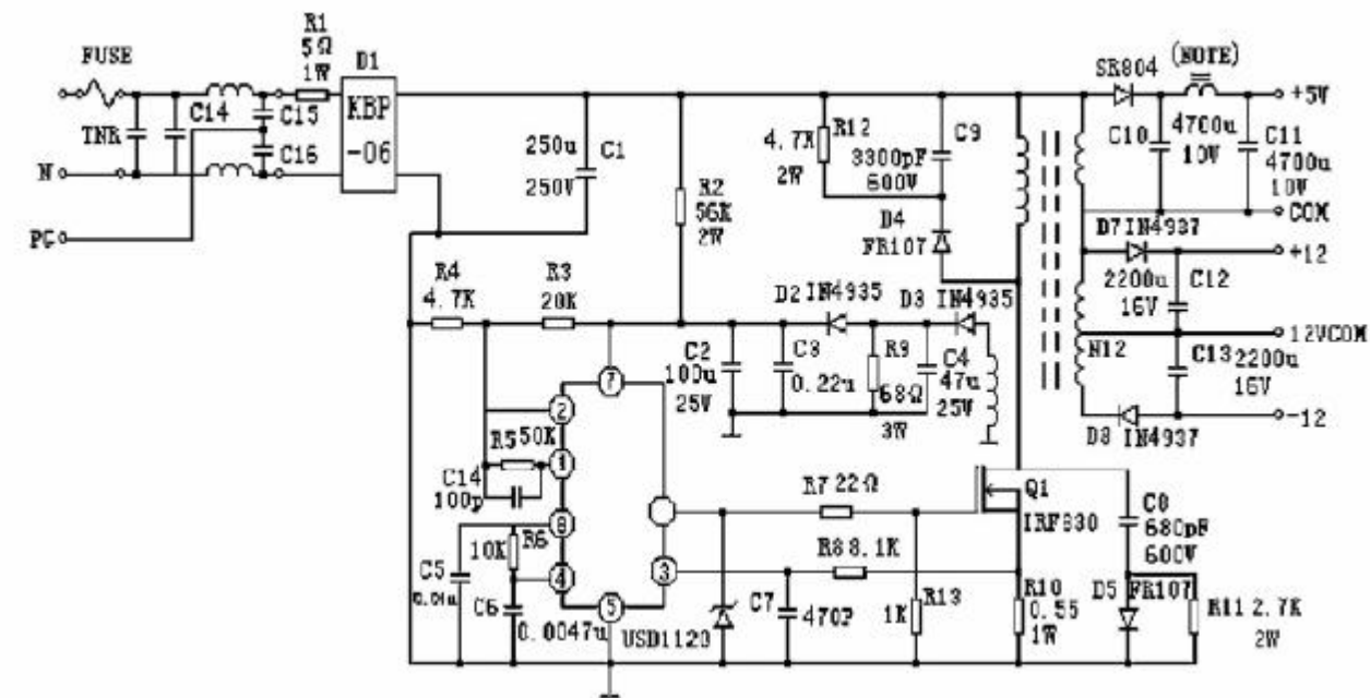
应用电路图
