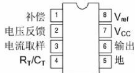
管脚连接图
