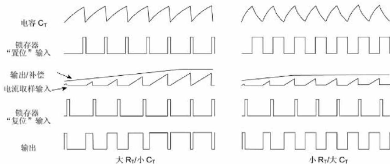
图 18. 时序图
