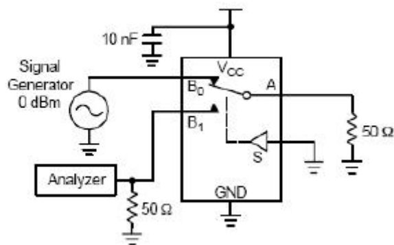
图 5 串扰
