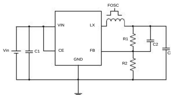
测试电路 2
