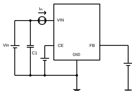
测试电路 3
