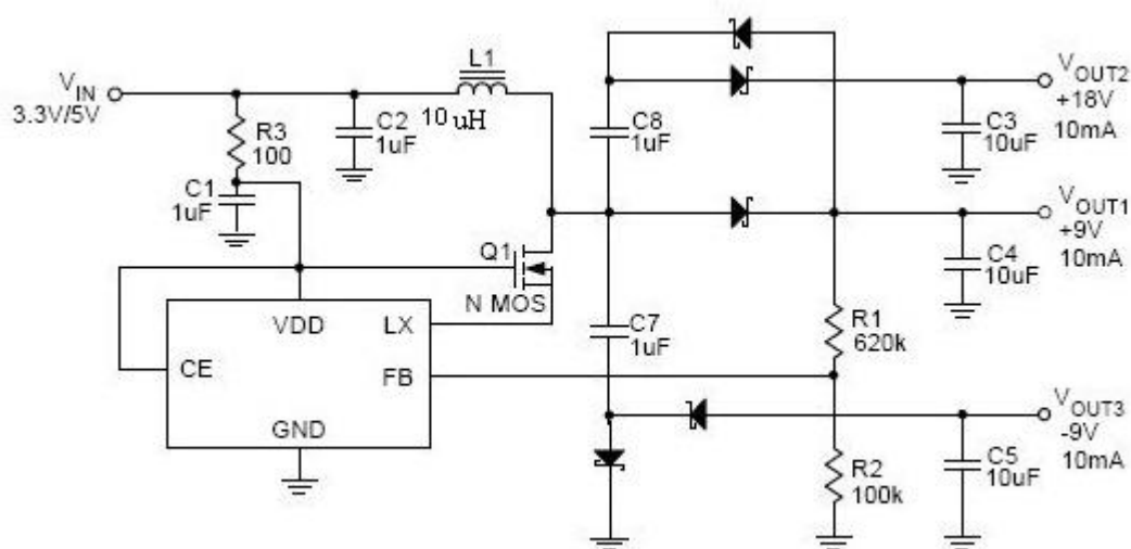
电路 2 JTML2266 多路输出的应用
