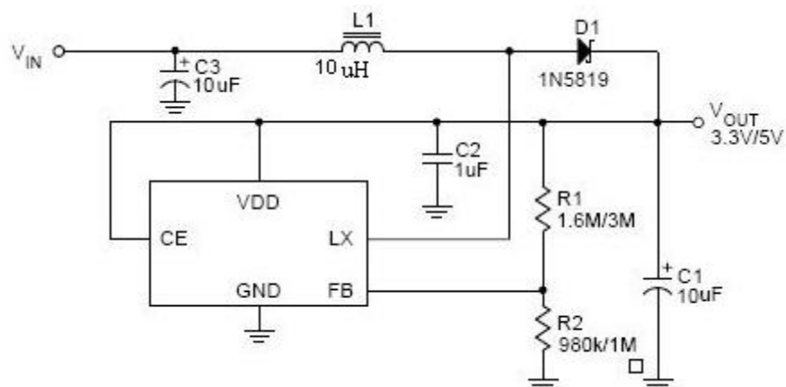
电路 1 JTML2266 在便携式仪器中的典型应用
