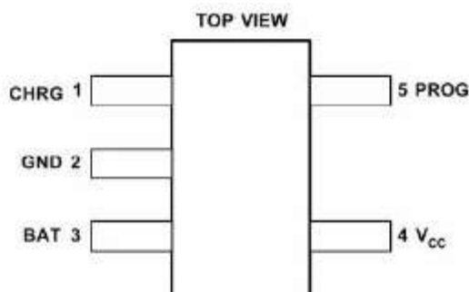
图 1.封装
