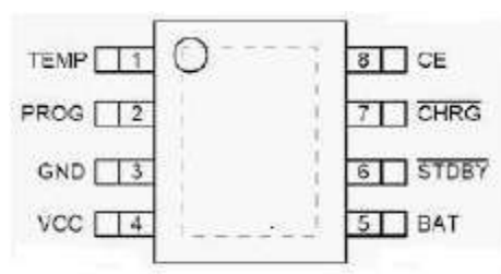
图 4. SLM6150 引脚封装图
