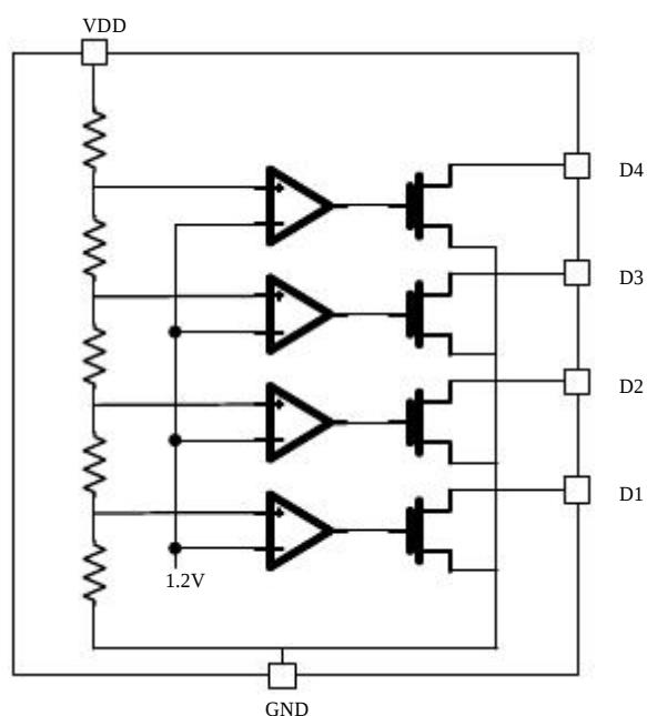
功能框图
