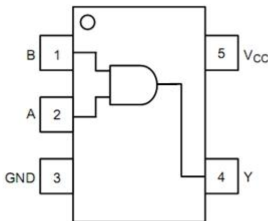
图 1 脚位图
