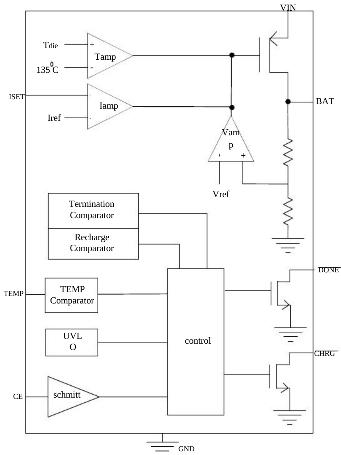
图 2 功能框图
