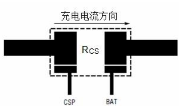
图 4 充电电流的检测
