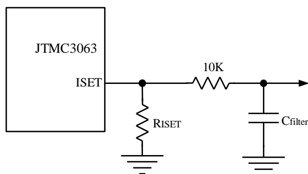
图7 隔离ISET管脚的电容负载
