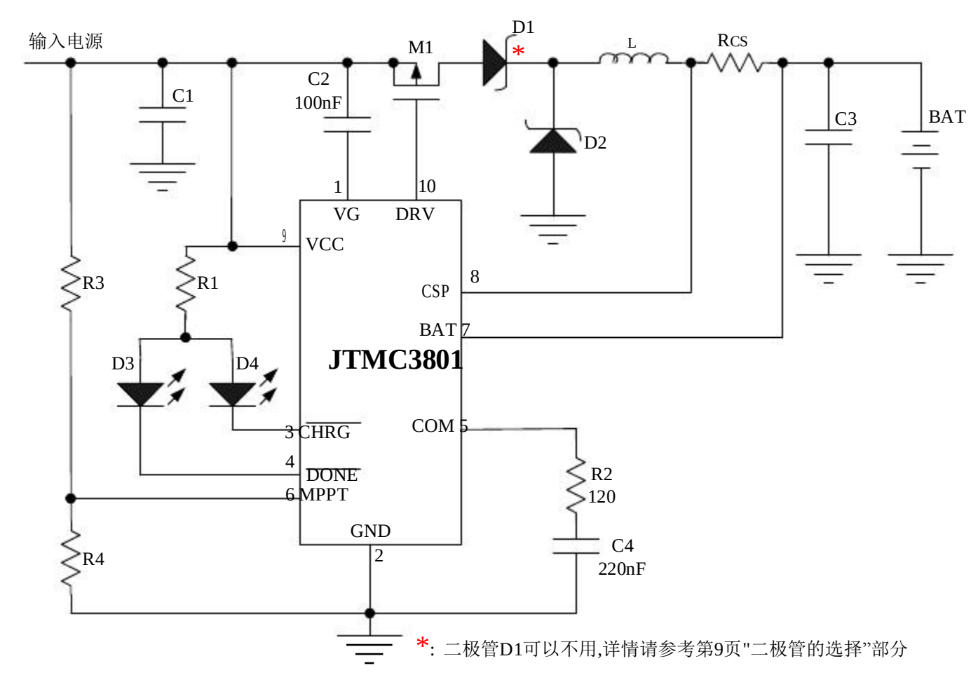
图 1 典型应用电路
