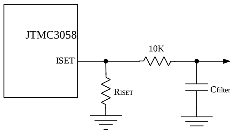
图7 隔离ISET管脚的电容负载
