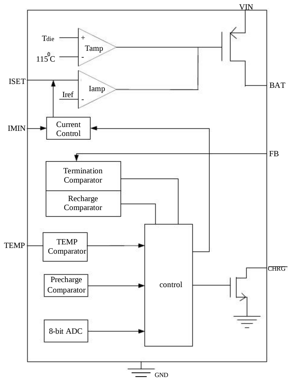
图 2 功能框图
