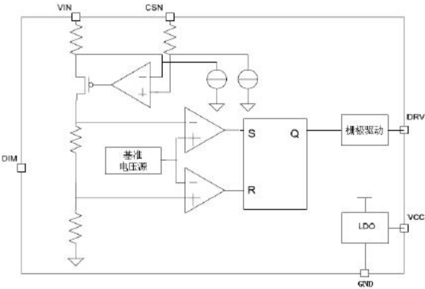
图 2 功能框图
