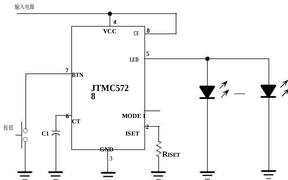
图 5 JTMC5728 驱动并联发光二极管(LED)
