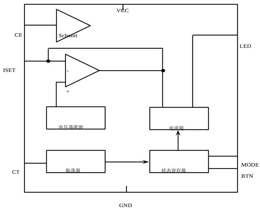
图 4 功能框图
