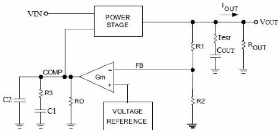
图 2 频率响应相关电路
