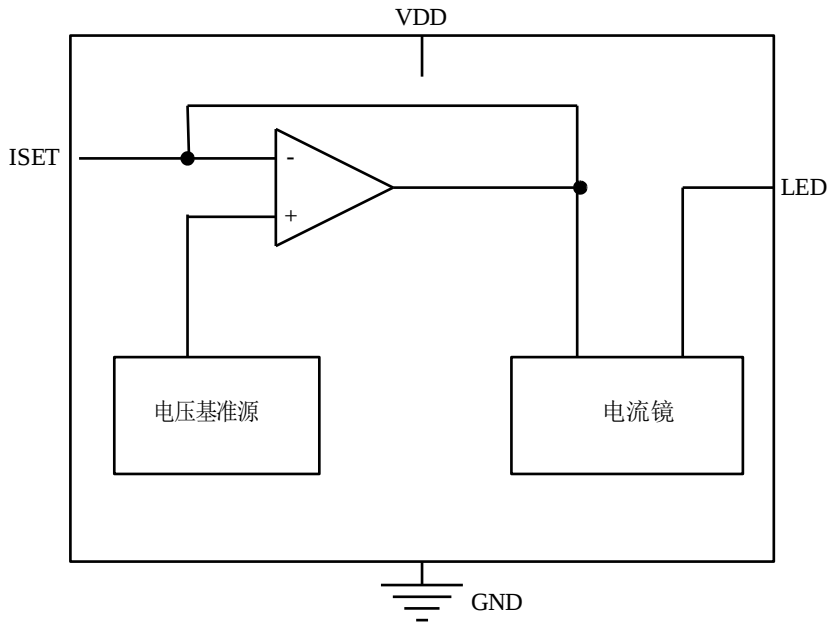
图 2 功能框图
