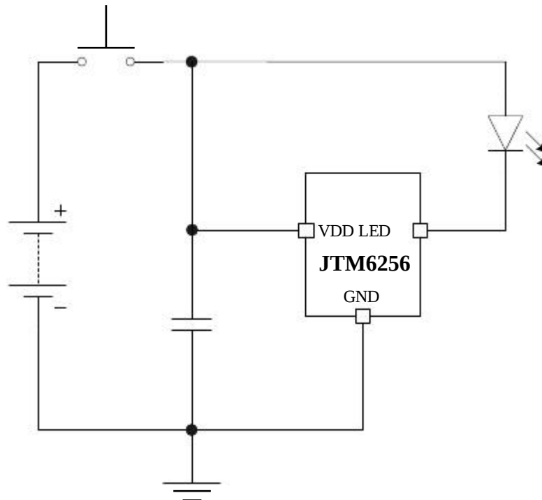
图 1：JTM6256 典型应用电路图
