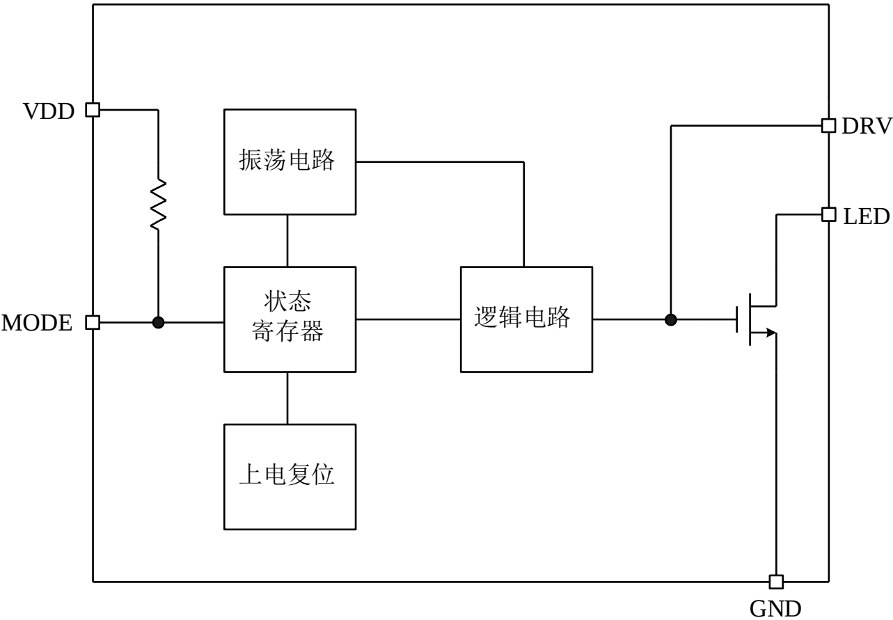
图 2: JTM6256 内部电路方框图
