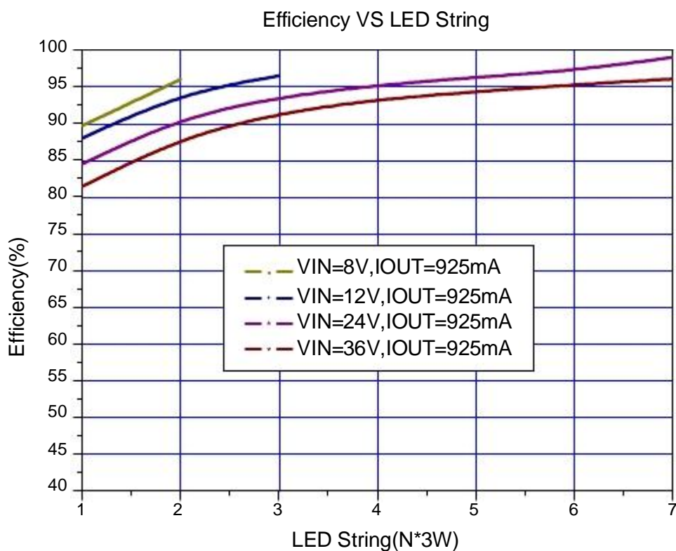
图18. JTMX3787系统效率曲线
