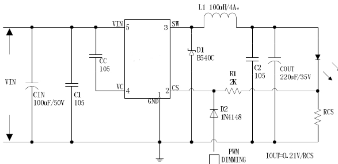
图 19. JTMX3787 系统参数测量电路（PWM DIMMING）
