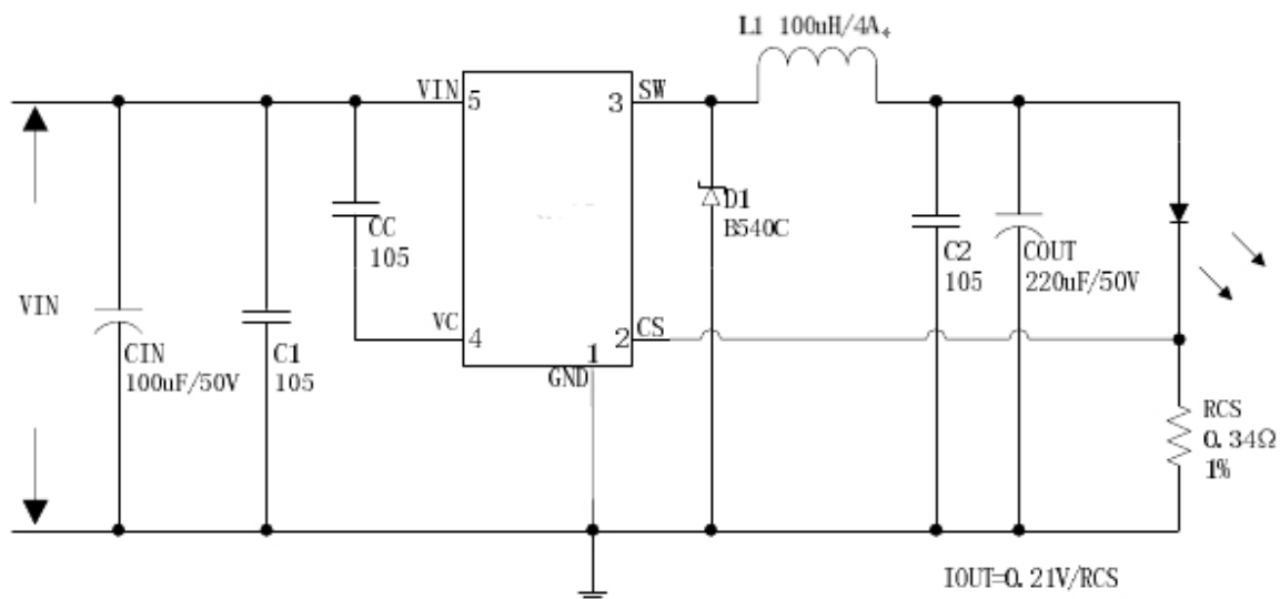
图 15. JTMX3787 系统参数测量电路 (VIN=8V~36V, IOU=615mA)
