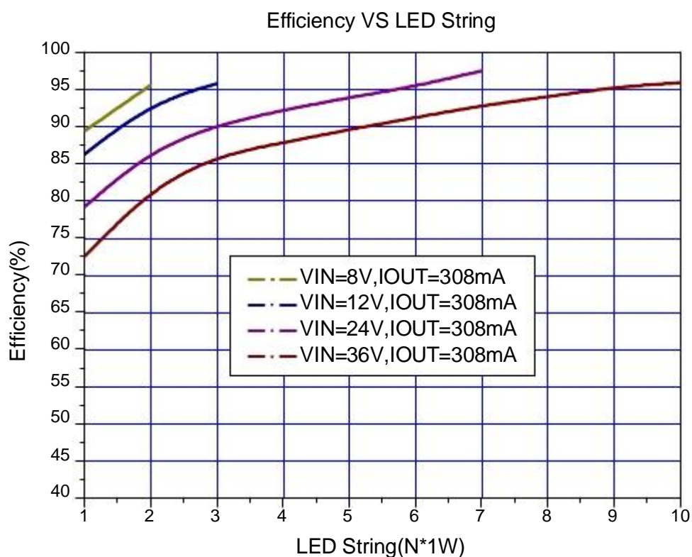
图14. JTMX3787系统效率曲线
