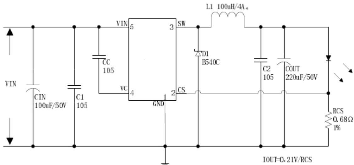
图 13.JTMX3787 系统参数测量电路 (VIN=8V~36V,IOUT=308mA)
