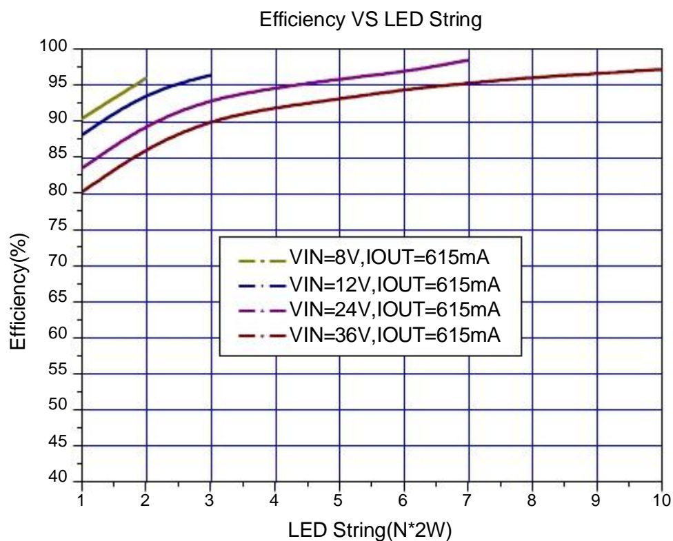
图16. JTMX3787系统效率曲线
