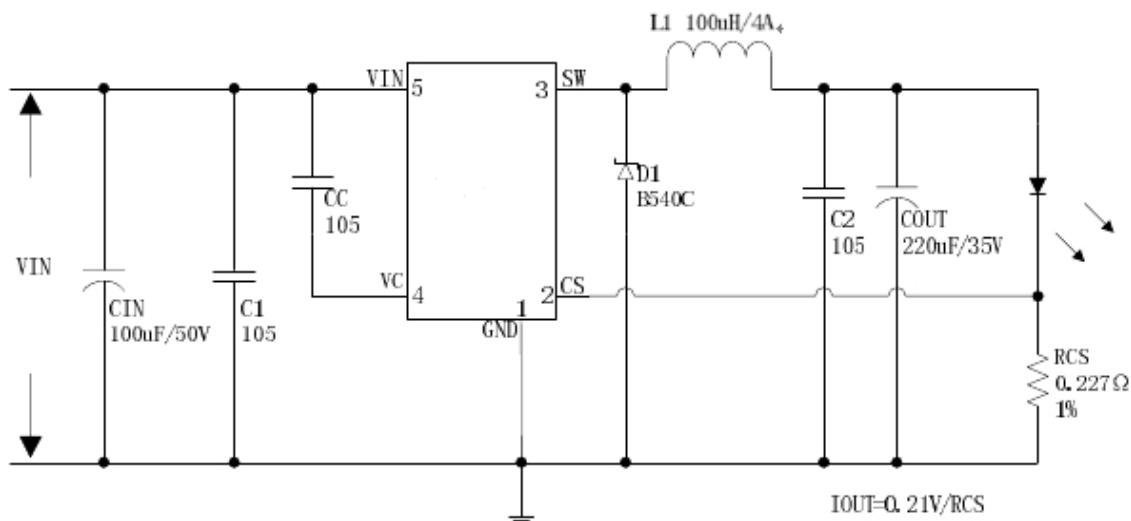
图 17. JTMX3787 系统参数测量电路 (VIN=8V~36V, IO UT =925mA)
