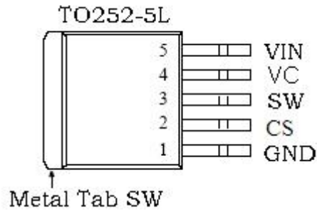
图 2. JTMX3787 引脚配置
