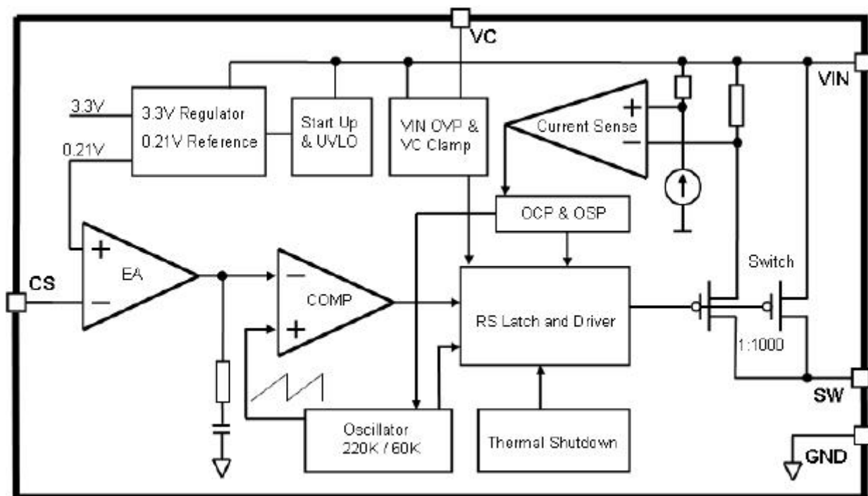
图 3. JTMX3787 方框图
