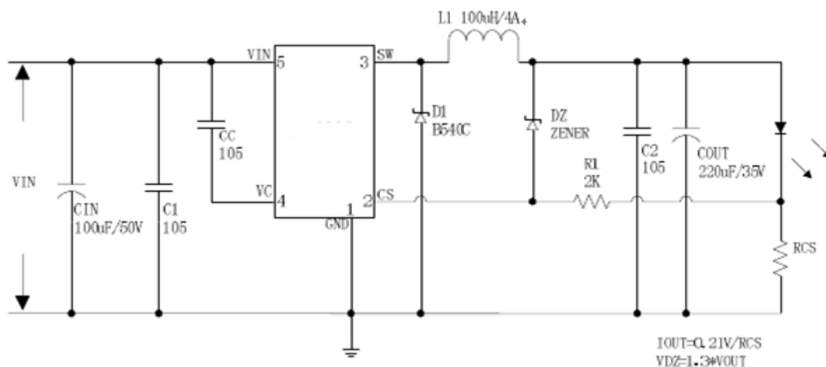
图20. JTMX3787系统参数测量电路（LED OVP）
