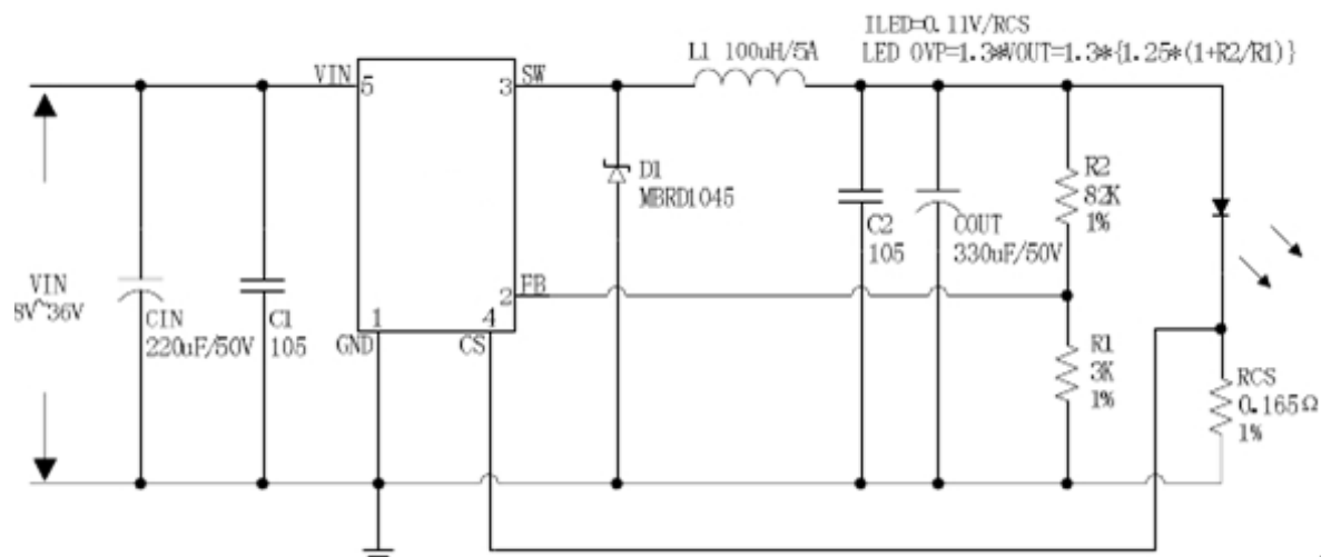
图 22. JTMX4985 系统参数测量电路 (VIN=8V~36V, IO UT =660mA)
