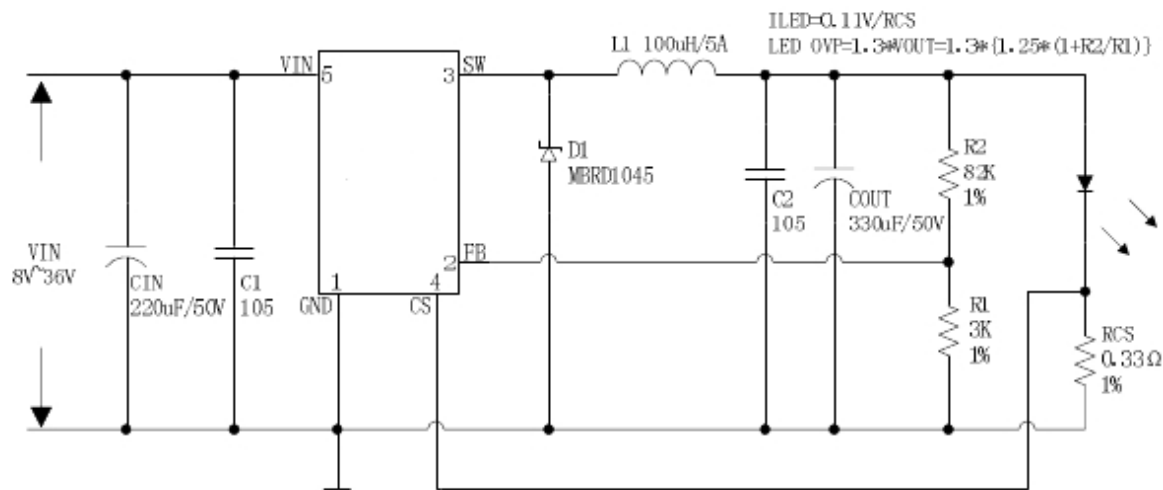
图 20.JTMX4985 系统参数测量电路 (VIN=8V~36V,IOUT=330mA)
