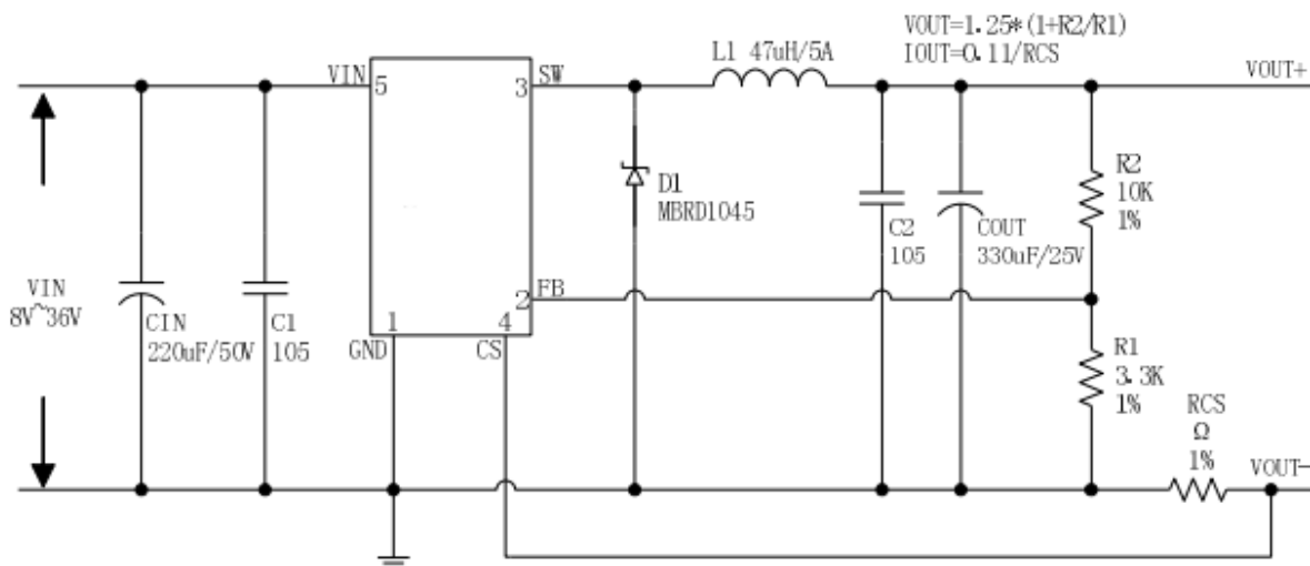
图 4. JTMX4985 系统参数测量电路
