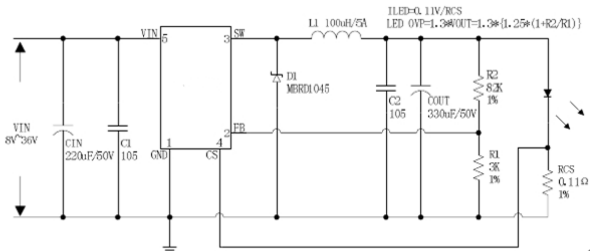
图 24. JTMX4985 系统参数测量电路 (VIN=8V~36V, IO UT =1000mA)
