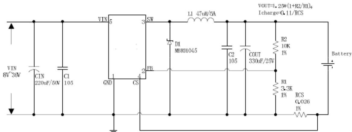
图 6.JTMX4985 系统参数测量电路 (VIN=8V~36V,VOUT=5V/0.1A~4.2A)
