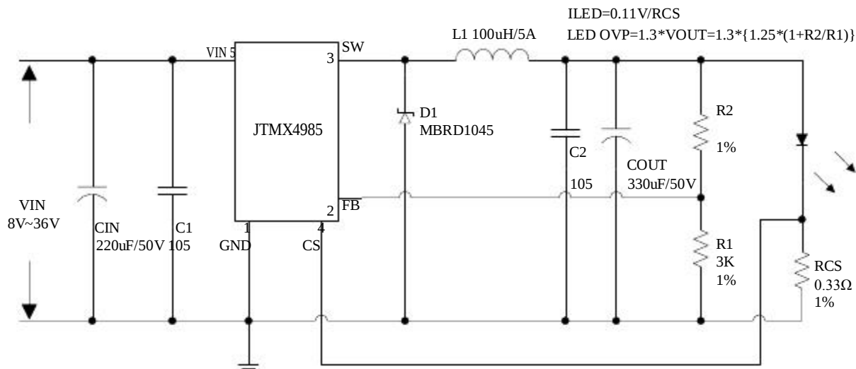
图 5.JTMX4985 系统参数测量电路(LED 恒流驱动)
