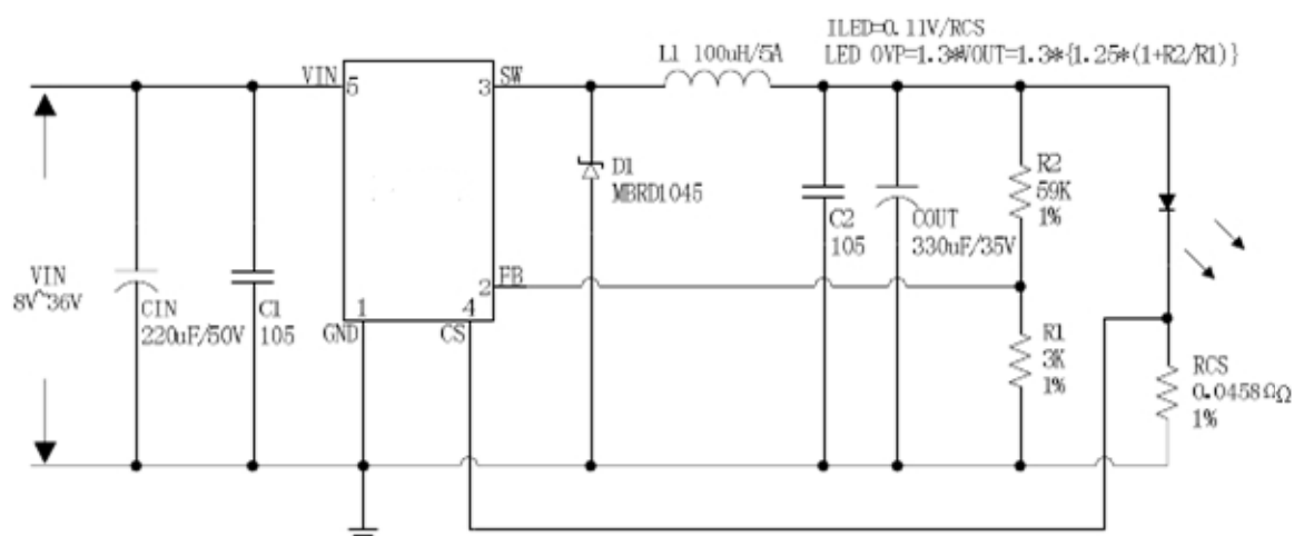
图 26. JTMX4985 系统参数测量电路 (VIN=8V~36V,IOUT=2400mA)
