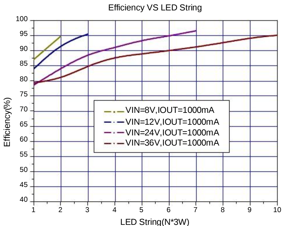
图25. JTMX4985系统效率曲线
