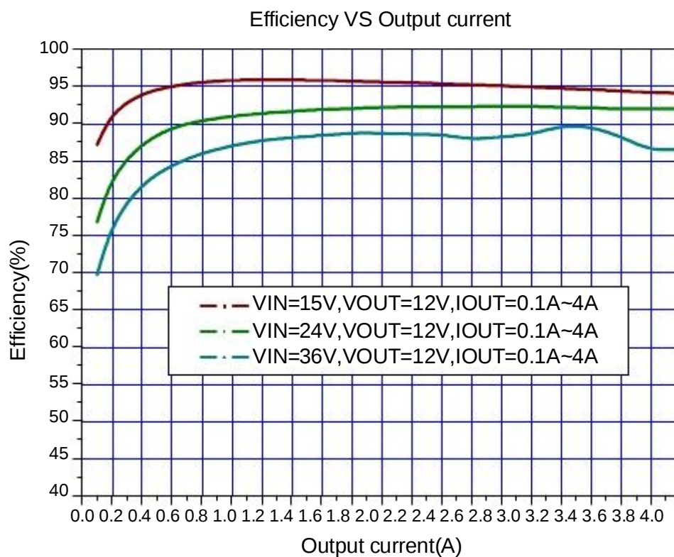
图19. JTMX4985系统效率曲线
