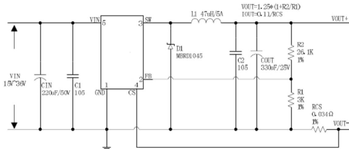
图 18.JTMX4985 系统参数测量电路 (VIN=15V~36V,VOUT=12V)
