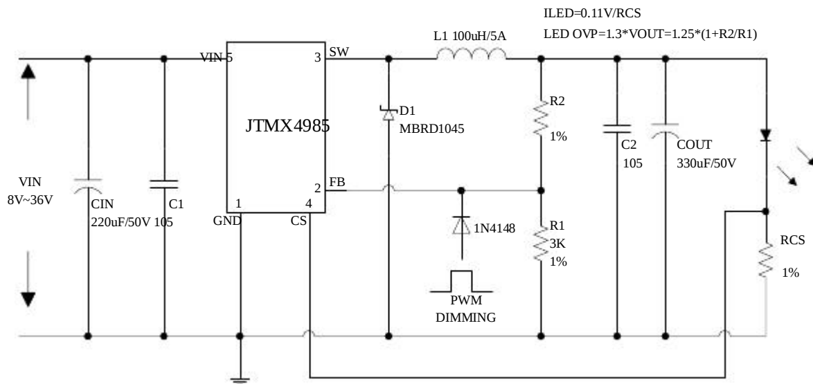
图 28. JTMX4985 系统参数测量电路
