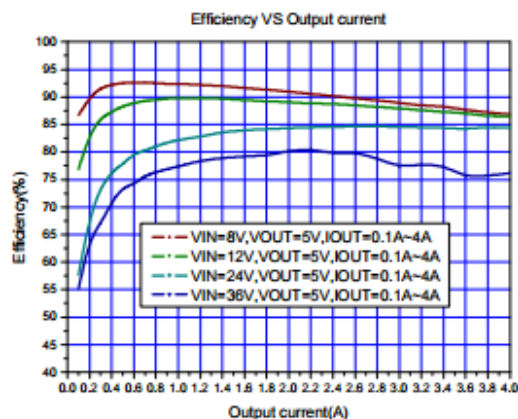
图 8. 效率曲线
