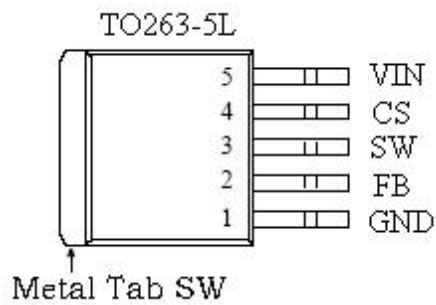
图 2. JTMX4985 引脚配置
