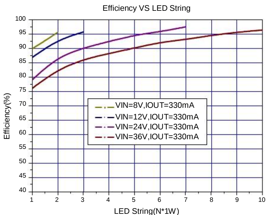
图21. JTMX4985系统效率曲线
