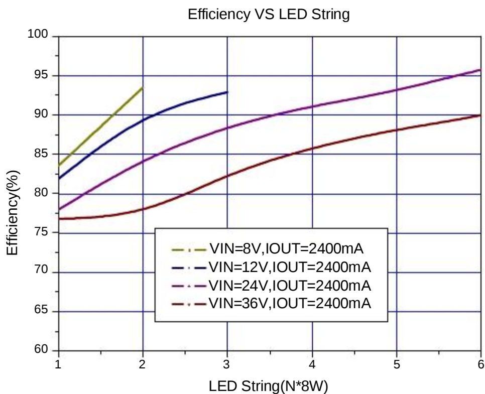
图27. JTMX4985系统效率曲线
