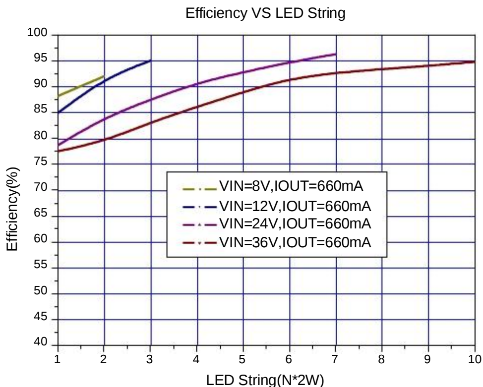
图23. JTMX4985系统效率曲线
