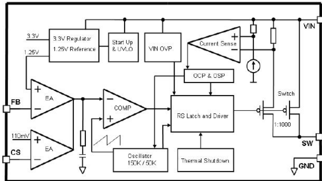
图 3. JTMX4985 方框图
