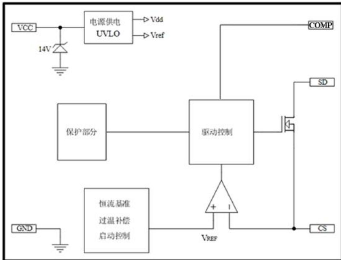
芯片内部方框图
