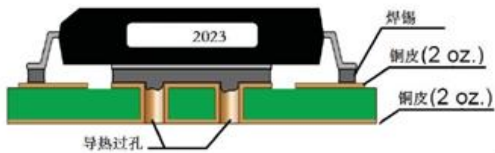
PCB 剖面图
